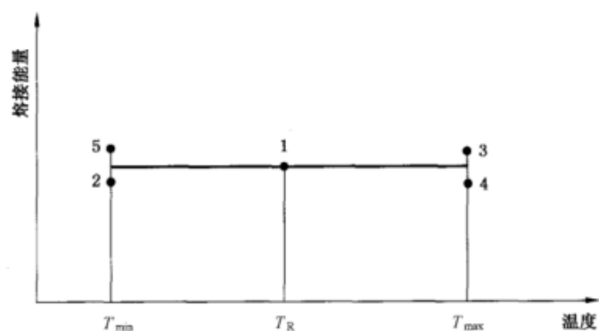
图 B.2 能量恒定的曲线
